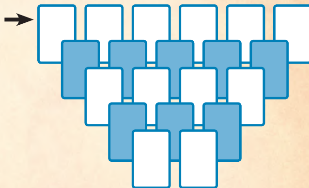
Епоха 3
