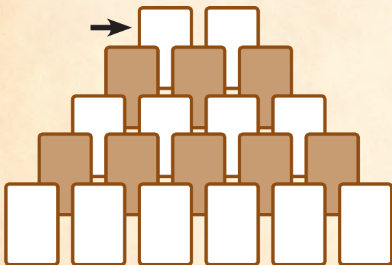
Епоха 1
